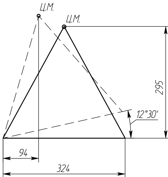
Рисунок 1- Схема устойчивости электронасосного агрегата типа 2К80-65-160.
